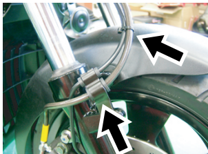
ブレーキホースをボトムケース部のホースクランプに固定し、タイラップ150mmでスピードメーターハーネスを固定します
