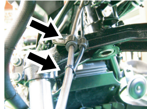
ブレーキホースをステム部のホースクランプに固定し、タイラップ150mmでスピードメーターハーネスを固定します
