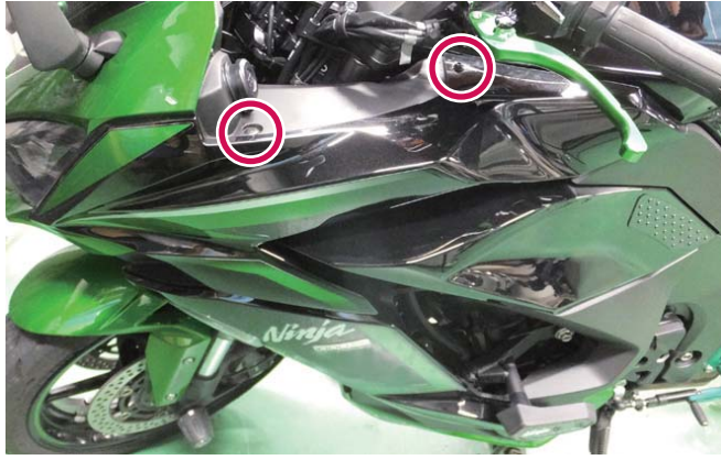
2-1. ボルト・クリップを取り外します。
