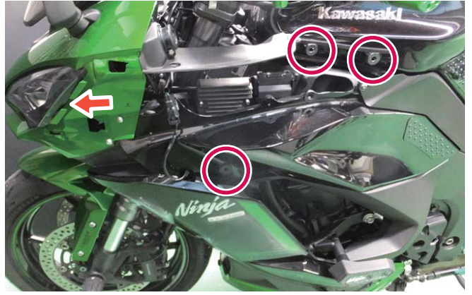
2-2. ボスを抜き、前方へカウルを取り外します。
