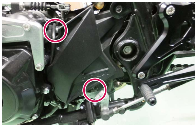
2-7. スプロケットカバーを取り外します。
