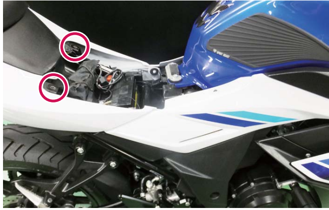
2-1. シートを取り外します。(ボルト2ヶ所)
