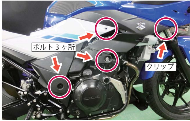
2-5. フレームカウルを取り外します。(4ヶ所)
